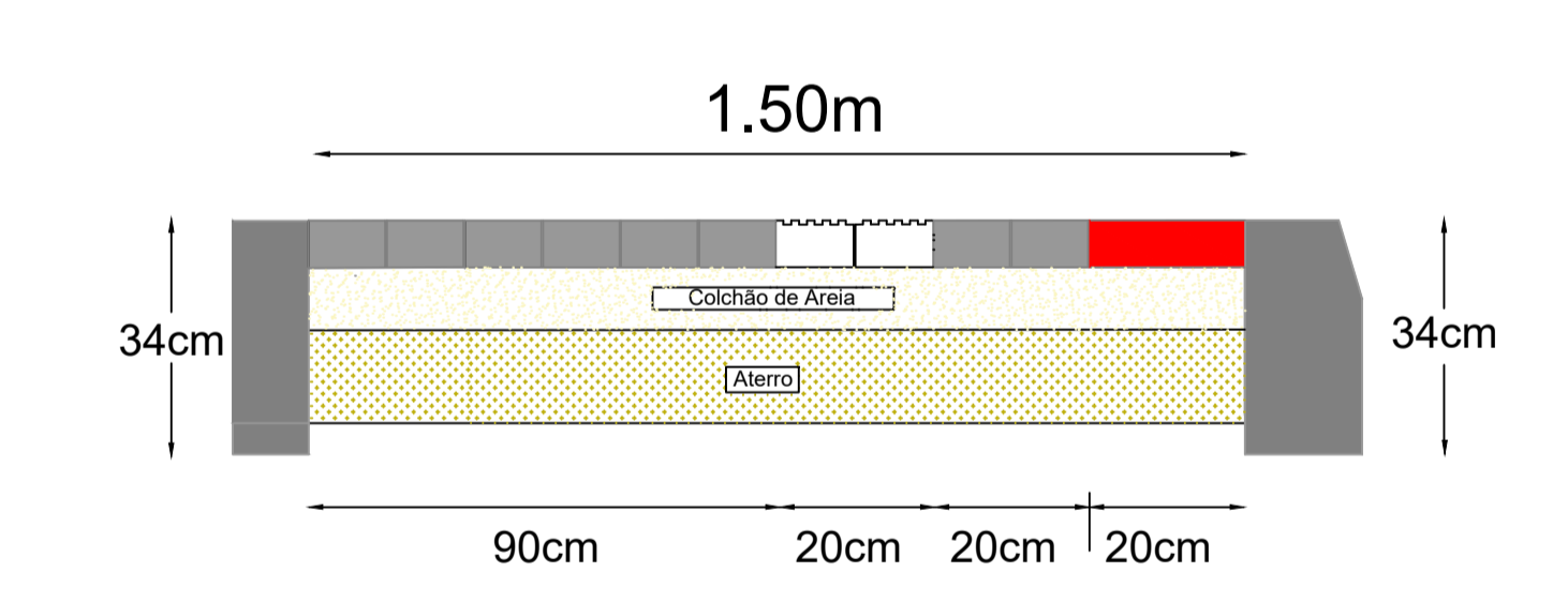
DETALHE CALÇADA SEM ESCALA
