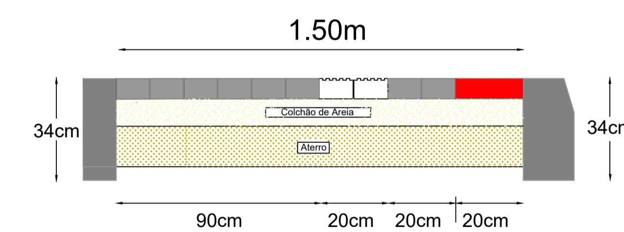
DETALHE CALÇADA SEM ESCALA
