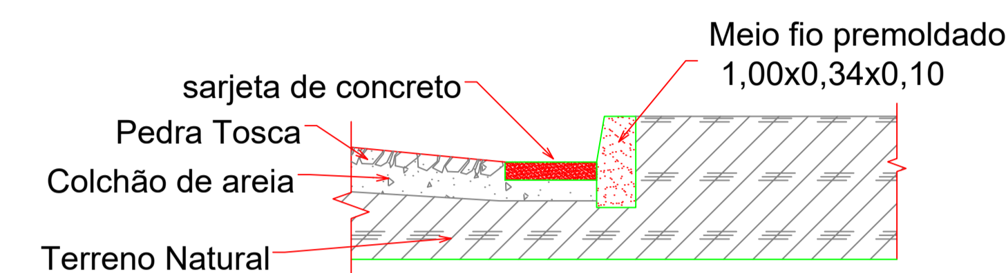
DETALHE SARJETA SEM ESCALA
