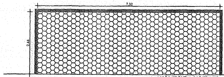
VISÃO FRONTAL DAS TRAVES ESC.: 1/20
