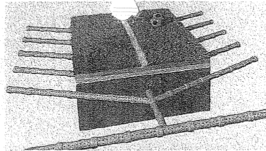
DETALHE PERFIL - DRENAGEM DO CAMPO SEM ESCALA
