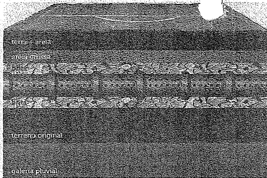
VISTA TRANSVERSAL - DRENAGEM SEM ESCALA
