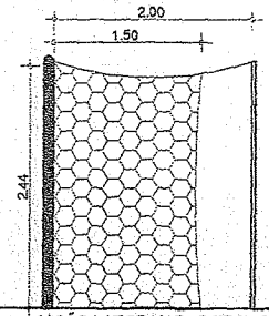
VISÃO LATERAL DAS TRAVES ESC.: 1/20
