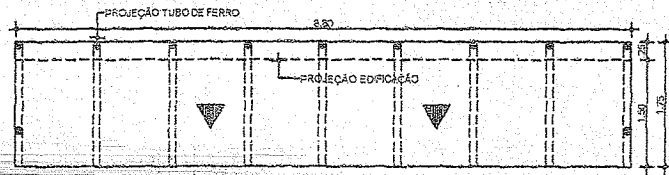
ESTRUTURA: METÁLICA COBERTA: POLICARBONATO TRANSPARENTE PLANTA BAIXA - COBERTA ESC.: 1/25
