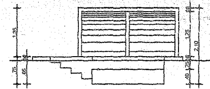
CORTE AB ESC.: 1/25
