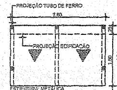
ESTRUTURA: METÁLICA COBERTA: POLICARBONATO TRANSPARENTE PLANTA BAIXA - COBERTA ESC.: 1/25
