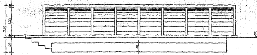
CORTE AB ESC.: 1/25
