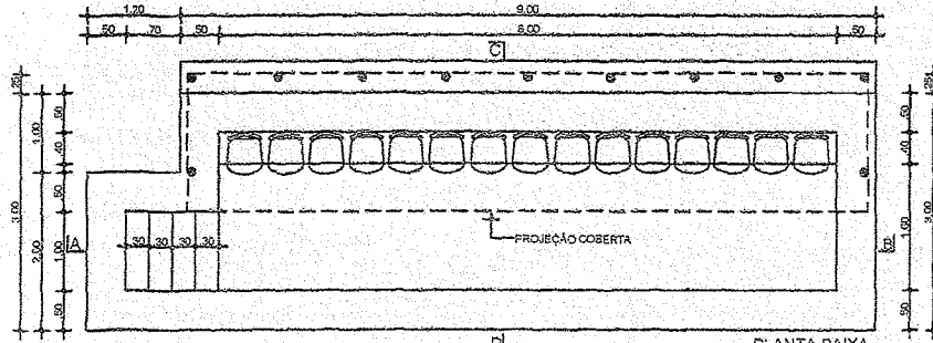
PLANTA BAIXA ESC.: 1/25
