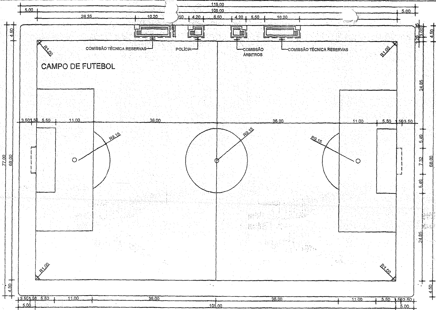
PLANTA BAIXA ESC.: 1/150
