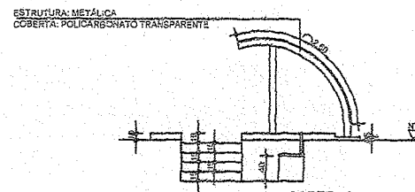
CORTE CD ESC.: 1/25
