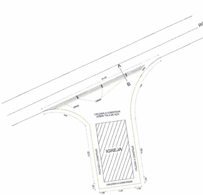
PLANTA BAIXA
