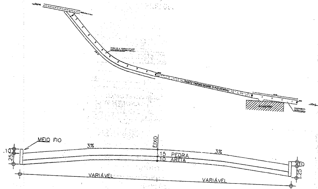
SEÇÃO TRANSVERSAL PADRÃO SEM ESCALA
