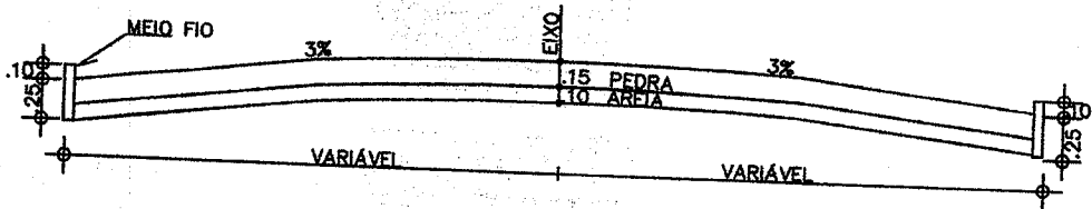
SEÇÃO TRANSVERSAL PADRÃO SEM ESCALA
